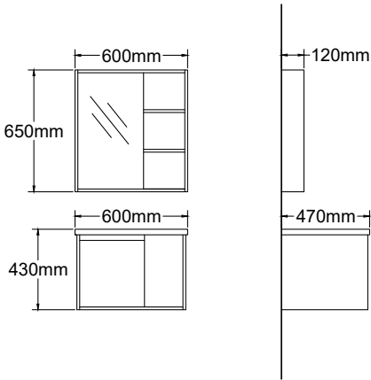
T-9100 主柜 /Main Cabinet : 600x470mm 镜柜 /Mirror Cabinet : 600x650mm 陶瓷盆 /Wash Basin 材质 /Plywood
