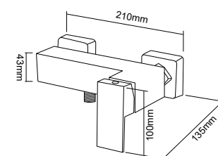
DT-1115 淋浴龙头 Shower faucet 材料 /Material: A 级铜 /Brass
