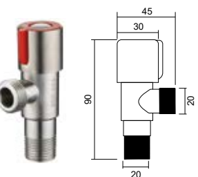
DJF-018BR 角阀 Angle valve 材料 /Material: 不锈钢 /SUS304
