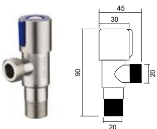
DJF-017BR 角阀 Angle valve 材料 /Material: 不锈钢 /SUS304
