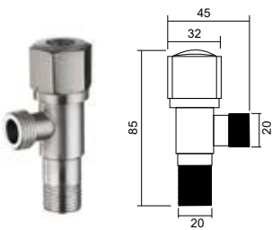
DJF-010BR 角阀 Angle valve 材料 /Material: 不锈钢 /SUS304
