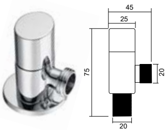
JF-046 角阀 Angle valve 材料 /Material: A 级铜 /Brass
