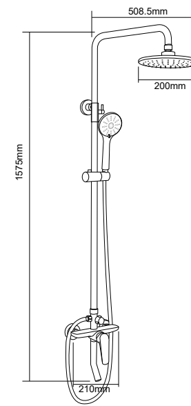
DT-1911 淋浴套件 Shower set 材料 /Material: A 级铜 /Brass
