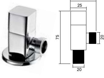
JF-047 角阀 Angle valve 材料 /Material: A 级铜 /Brass
