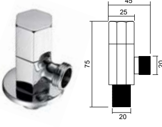
JF-012 角阀 Angle valve 材料 /Material: A 级铜 /Brass
