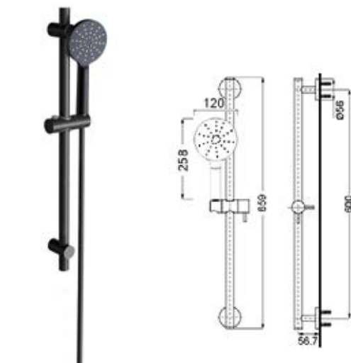
B-20B 升降杆 Sliding bar 材料 /Material: 不锈钢 /SUS304
