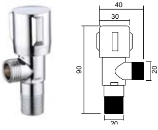
FJF-030 角阀 Angle valve 材料 /Material: A 级铜 /Brass
