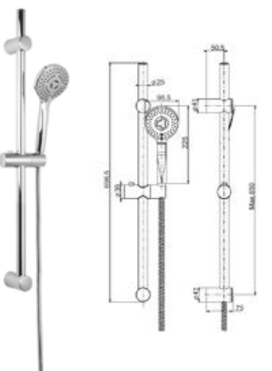
B-24 升降杆 Sliding bar 材料 /Material: 不锈钢 /SUS304
