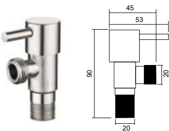
DJF-016BR 角阀 Angle valve 材料 /Material: 不锈钢 /SUS304
