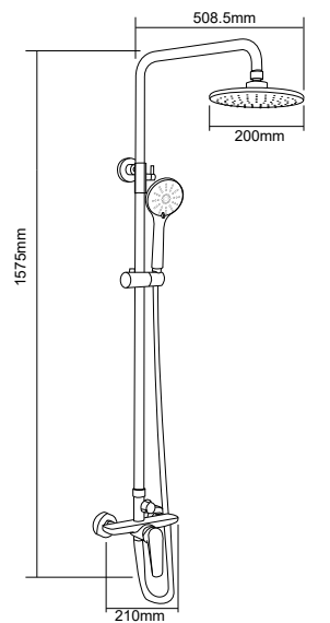
DT-1912 淋浴套件 Shower set 材料 /Material: A 级铜 /Brass
