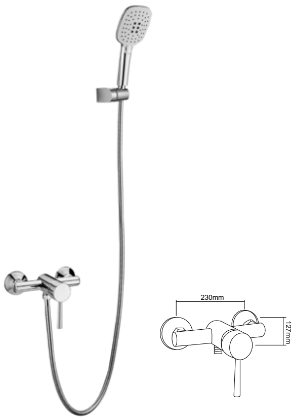
DT-5009 淋浴龙头 Shower faucet 材料 /Material: A 级铜 /Brass
