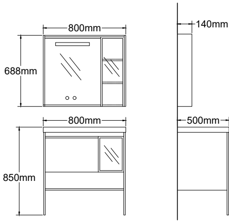
T-9042 LED+Anti-fog 主柜 /Main Cabinet : 800x500mm 镜柜 /Mirror Cabinet : 800x700mm 岩板 /Sintered Stone : Sky Black 材质 /Plywood
